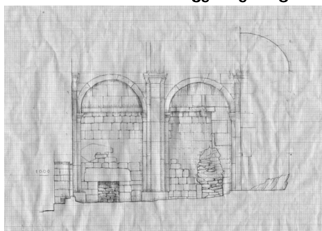
სურ. 4. მთავარი ეკლესიის წრილი ჩდრილოეთზე (არქ. შ. მელიქიძე)
