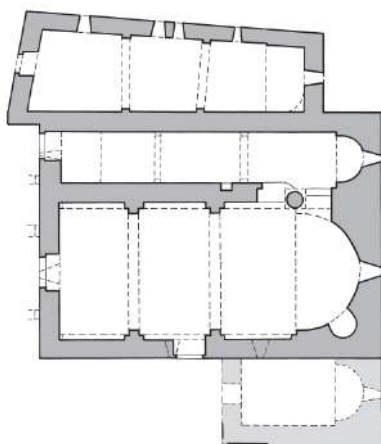
სურ. 2. ქუმის ეკლესია, გეგმა, ჭრილი
