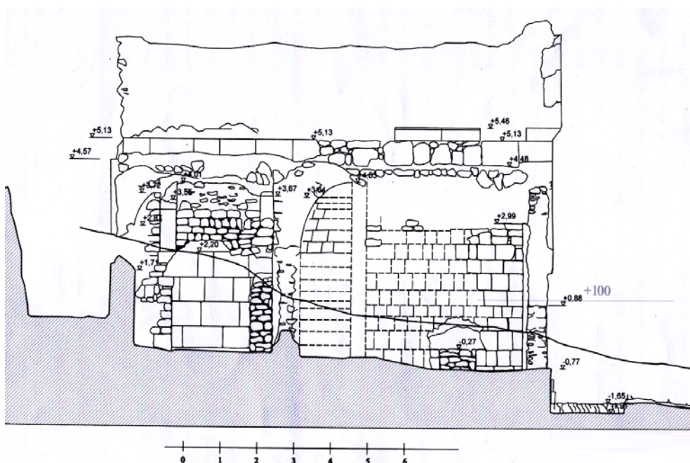
სურ. 4. ჯაყისმანის მონასტრის მოავარი ტაძარი. ტრილი ჩრდილოეთის მიმდებარე მცირე ეკლესიაზე (არქ. შ. მელიქიძე)
