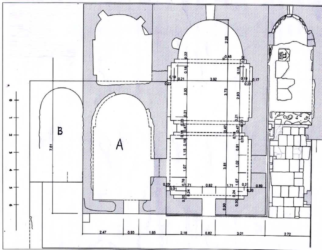
სურ. 3. ჯაყისმანის მონასტრის მთავარი ტაძარი და მიმდებარე ნაგებობები. გეგმა (არქ. შ. მელიქიძე)
