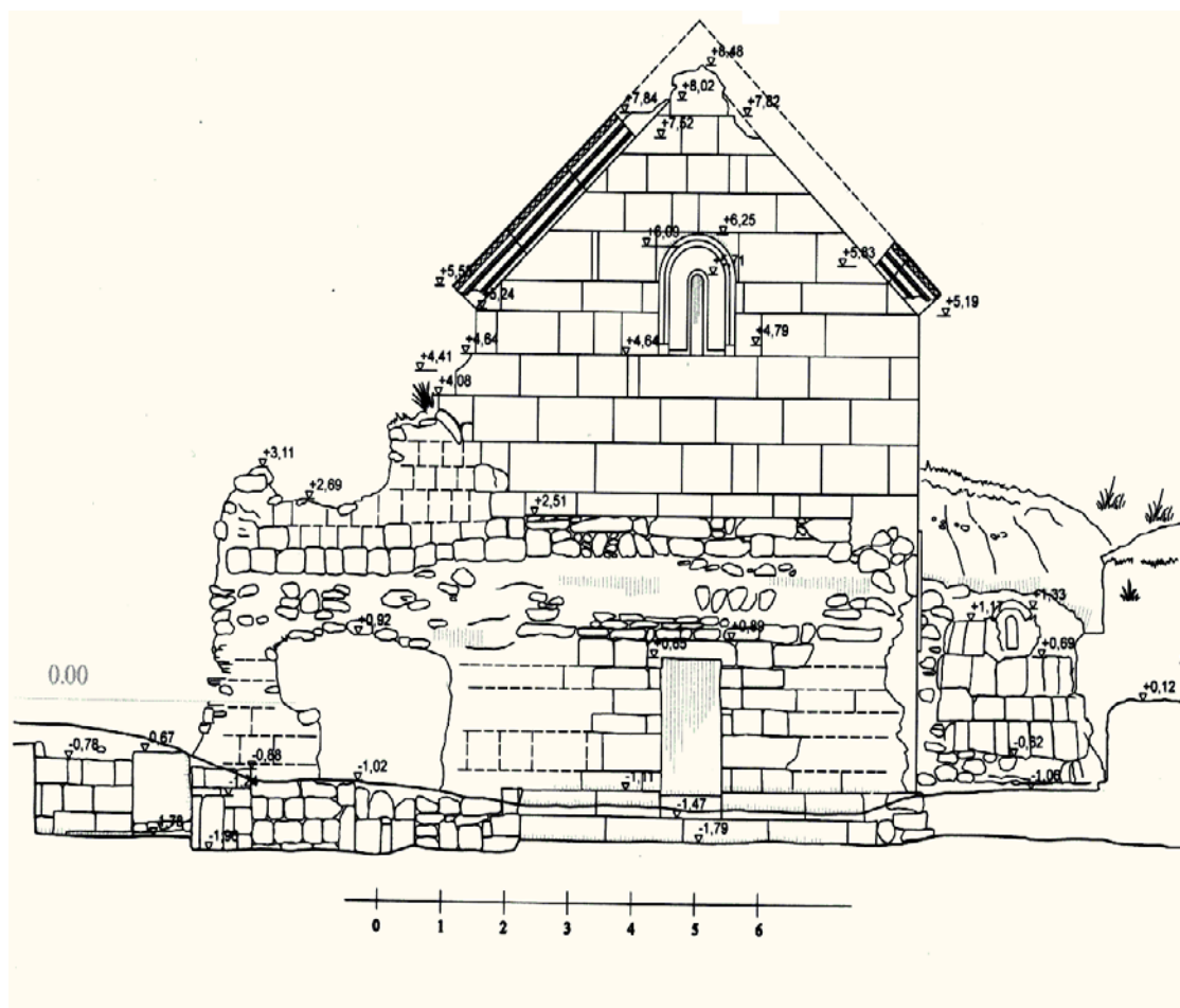
სურ. 9. ჯაყისმანის მონასტრის მთავარი ტაძარი. დასავლეთის ფასადი (არქ. შ. მელიქიძე)
