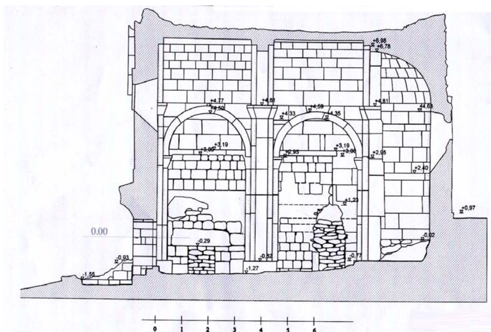
სურ. 6. ჯავისმანის მონასტრის მთავარი ტაძარი. ჭრილი ჩრდილოეთზე (არქ. შ. მელიქიძე)
