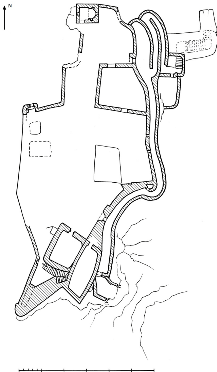
უზუნდერეს ციხის გეგმა. ავტორი გიორგი ბაგრატიონი
