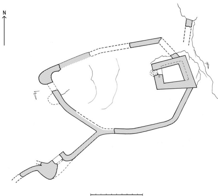
სურ. 6. ნიხაზის ციხის გეგმა. ავტორი გიორგი ბაგრატიონი
