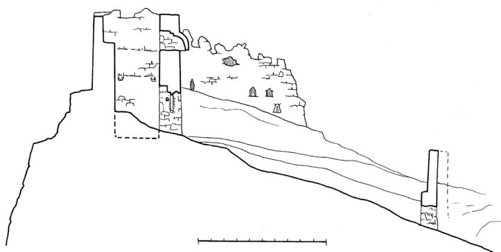
სურ. 7. ნიხაზის ციხის ჭრილი. ავტორი გიორგი ბაგრატიონი
